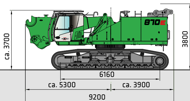
870 R Grundmaschine ohne Oberwagen-Geländer, ohne Gegengewicht, Transportgewicht ca. 66 t
